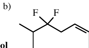
cis -5,5-difluoro-6-methyl-2-heptene or (Z) -5,5-difluoro-6-methyl-2-heptene
